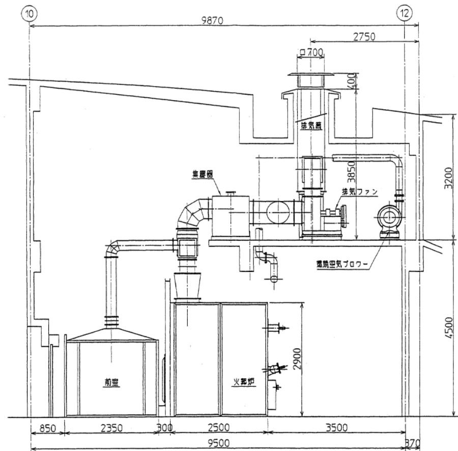
図4 断面図
