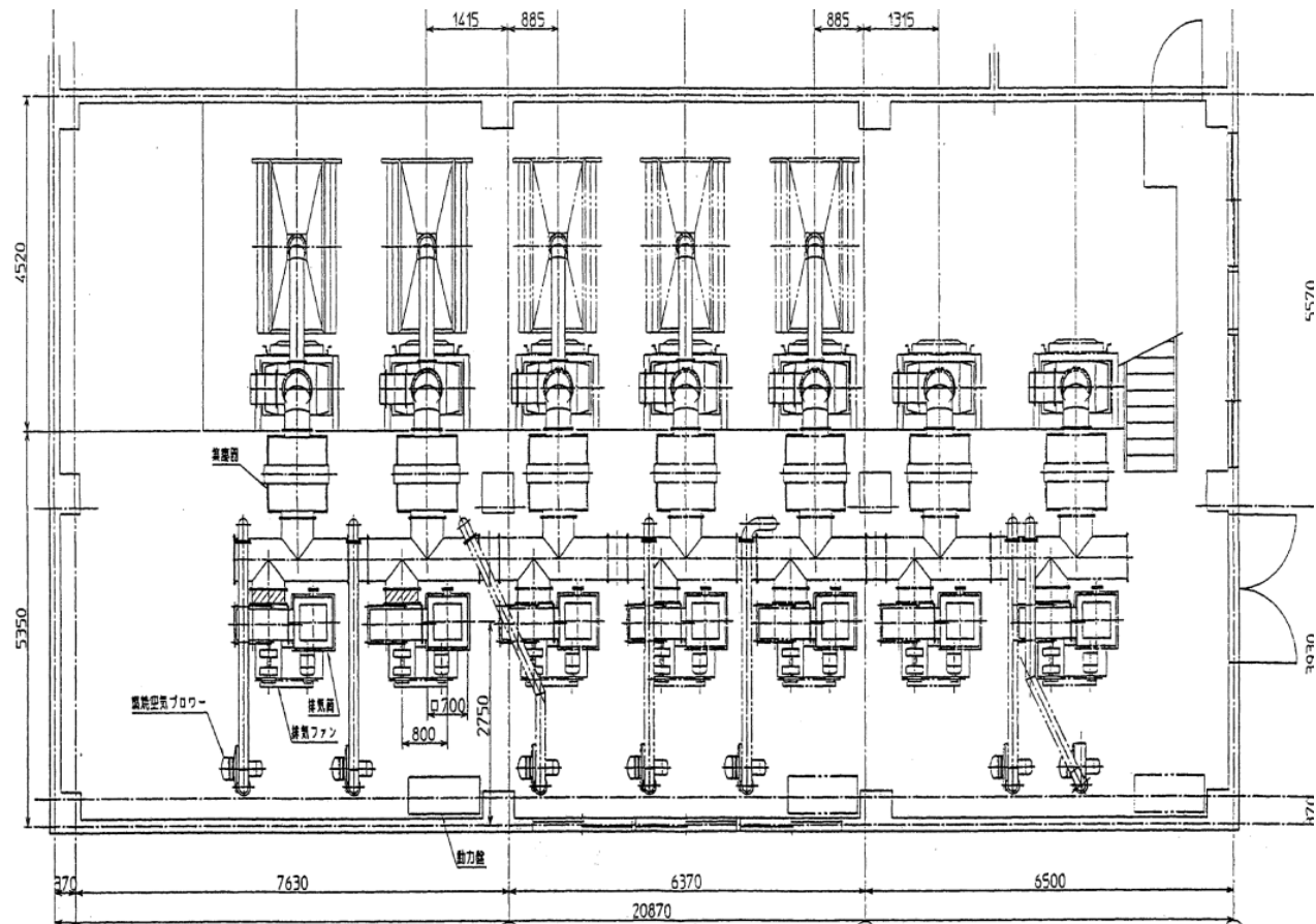
図3 2階機械室平面図
